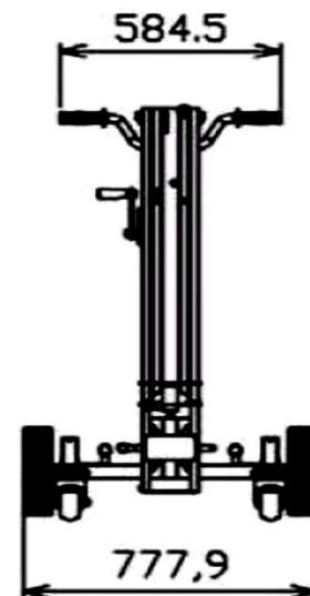
Roues à empattement réglable
